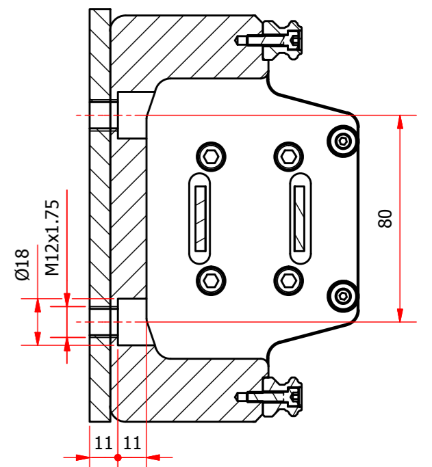
C-C (1:2)
