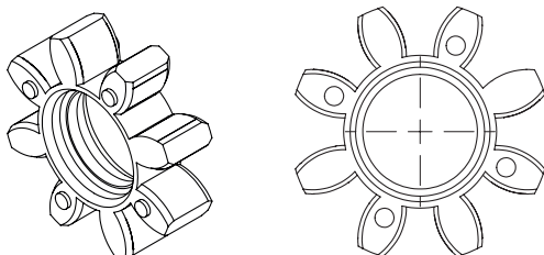
Fig. 16.34 Elastomer insert
